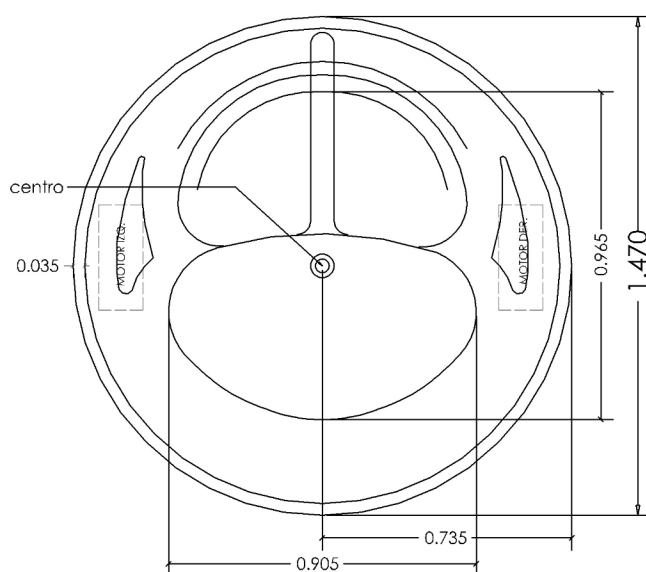
VISTA FRENTE
